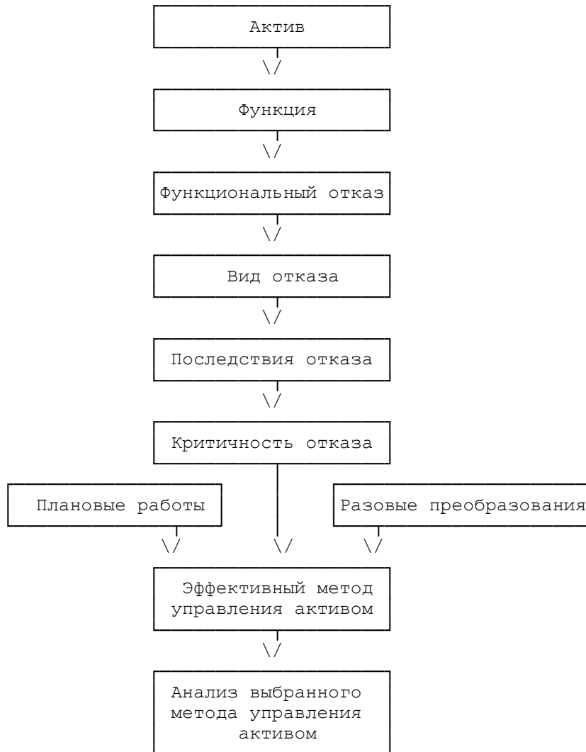
Рисунок А.1 - Блок-схема процесса НОТО
