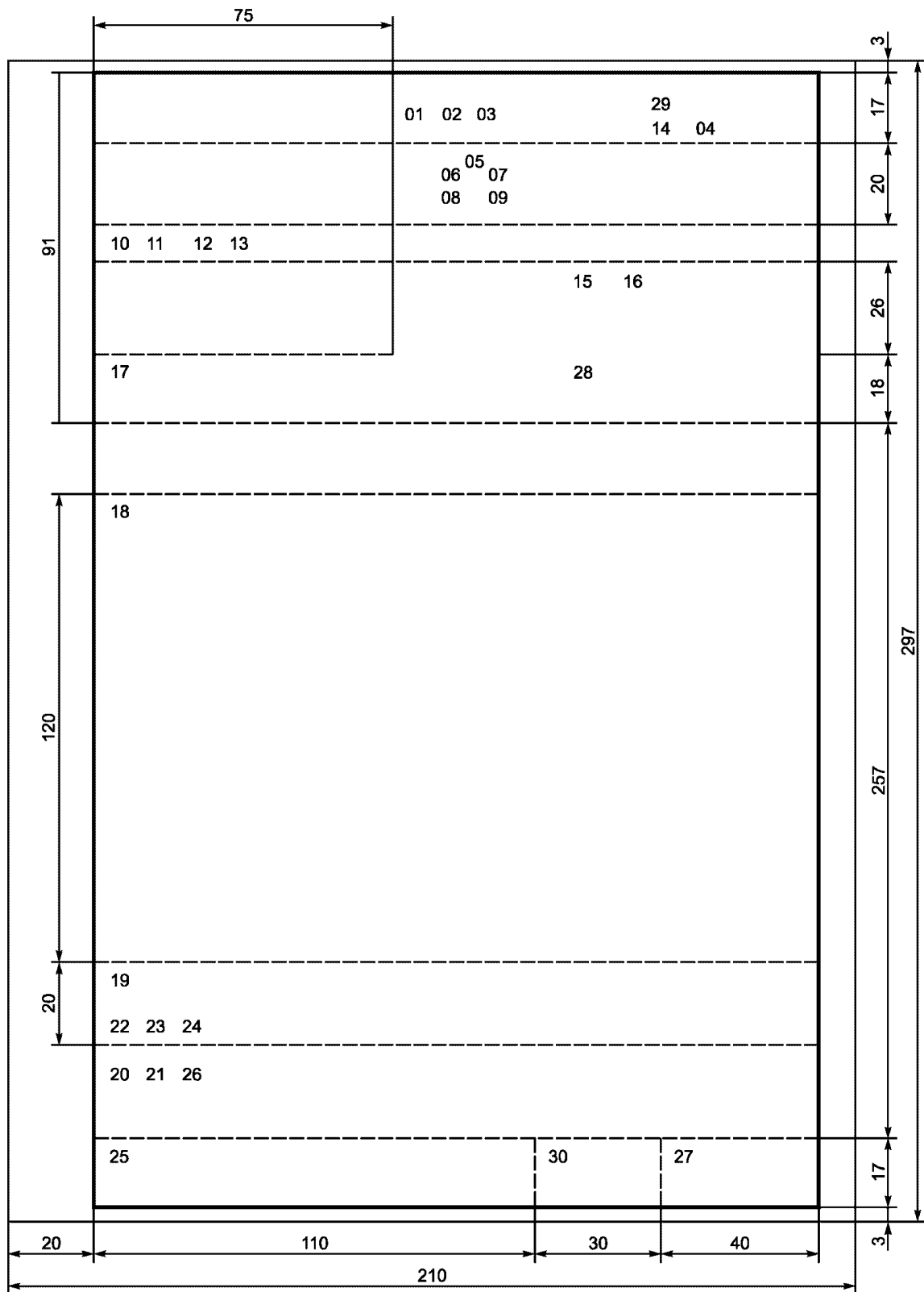
Рисунок Б.2 - Расположение реквизитов и границы зон
